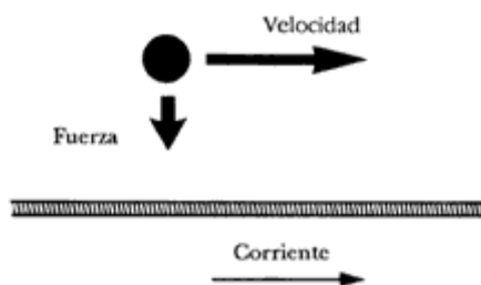
Figura 7. Una partícula cargada en movimiento resiente una fuerza de atracción (o repulsión) producida por una corriente eléctrica.
