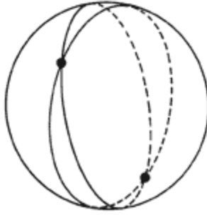
Figura 29. Las geodésicas son las curvas de menor longitud sobre una superficie curva.
