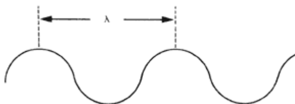
Figura 6. La longitud de onda.
