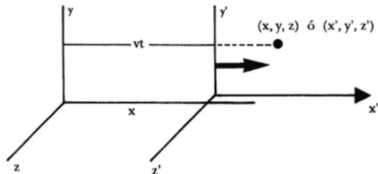
Figura 38. Dos sistemas de referencia en movimiento relativo.
